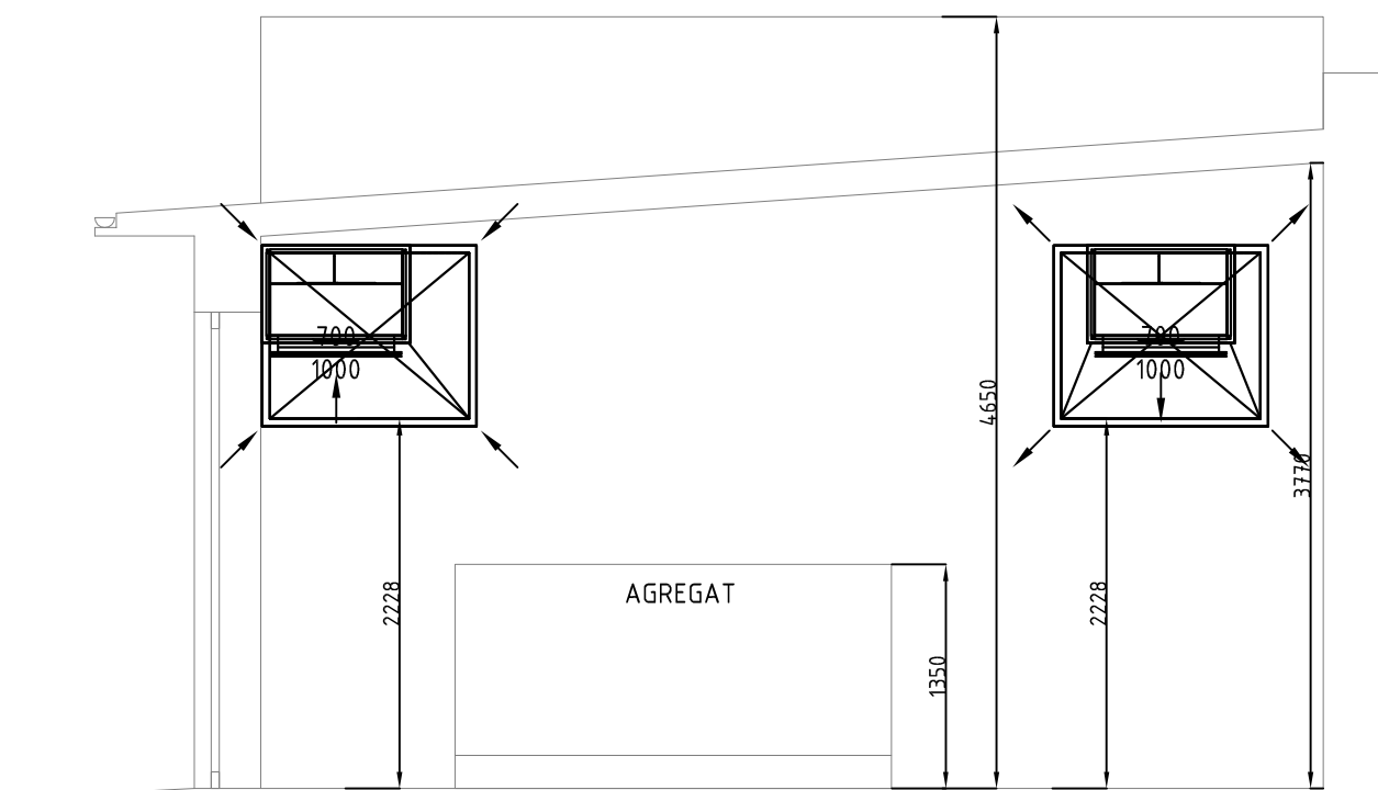
Przekrój A-A
