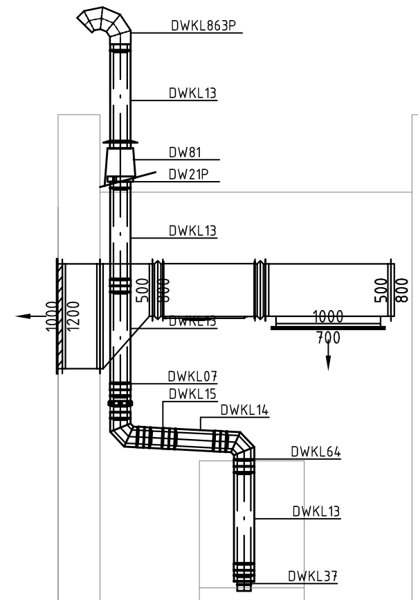
Przekrój B-B
